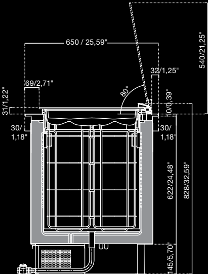
Vasca da incasso PANORAMA con riserva PANORAMA built-in tank with two levels of gelato tubs Cuve PANORAMA encastrable avec réserve Einbau-PANORAMA-Wanne für Gelato/Granita mit Vorrat Cuba PANORAMA empotrada con reserva
