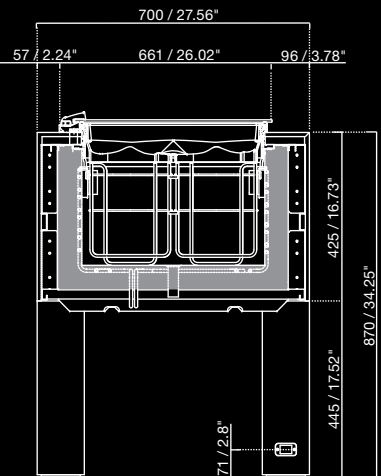
Tavolo BELLEVUE con vasca PANORAMA senza riserva BELLEVUE table with PANORAMA tank with one level of gelato tubs Table BELLEVUE avec cuve PANORAMA sans réserve BELLEVUE Theke mit PANORAMA-Wanne ohne Vorrat Mesa BELLEVUE con cuba PANORAMA sin reserva
