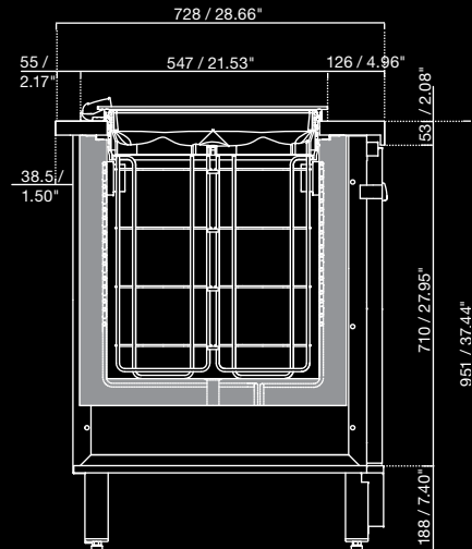
Banco PANORAMA con riserva PANORAMA counter with two levels of gelato tubs Comptoir PANORAMA avec réserve PANORAMA-Theke mit Vorrat Mostrador PANORAMA con reserva
