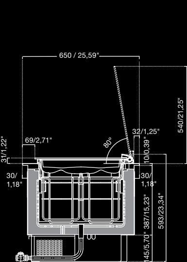
Vasca da incasso PANORAMA senza riserva PANORAMA built-in tank with one level of gelato tubs Cuve PANORAMA encastrable sans réserve Einbau-PANORAMA-Wanne für Gelato/Granita ohne Vorrat Cuba PANORAMA empotrada sin reserva
