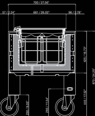
Tavolo BELLEVUE su ruote BELLEVUE table with castor wheels Table BELLEVUE avec roues pivotantes BELLEVUE Theke mit Rädern Mesa BELLEVUE con ruedas giratorias
